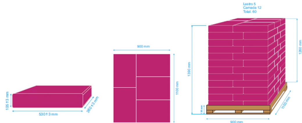
Montagem do pallet para produtos com 60 blocos/pallet.
