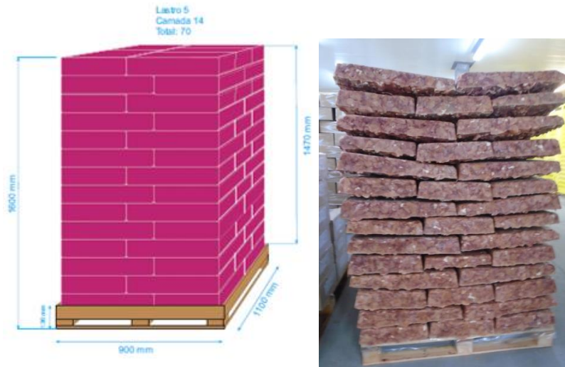
Montagem do pallet para produtos com 70 blocos/pallet.
